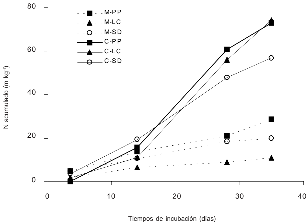
Figura 5. Nitrógeno mineralizado (M) y consumido (C) acumulados durante 35 días de incubación en un Molisol de Balcarce bajo pastura (PP) y agricultura continua bajo labranza convencional (LC) y siembra directa (SD).
