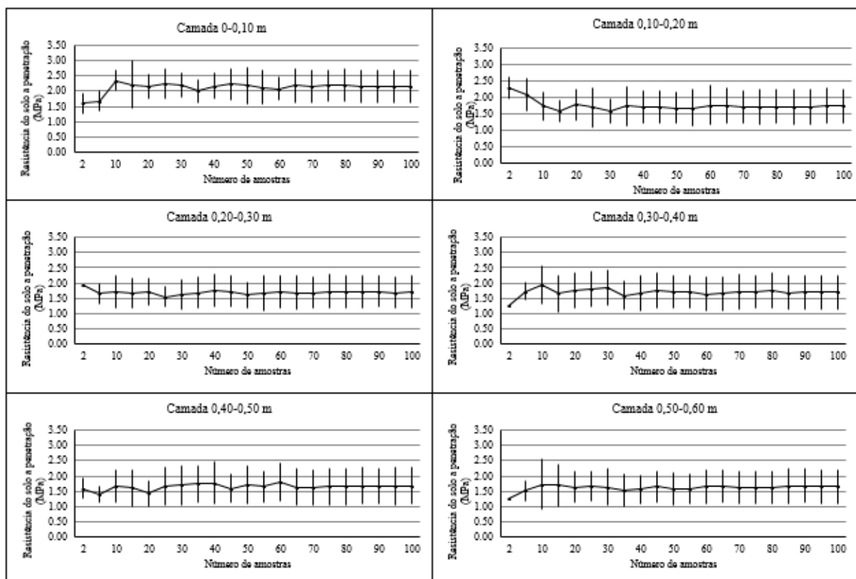
Figura 1. Variação dos valores de resistência do solo à penetração e os respectivos desvios padrões de um Latossolo Vermelho Distrófico sob mata nativa em função da população amostral(n), para área total de 19 ha. Palmeiras de Goiás, 02/2014.
