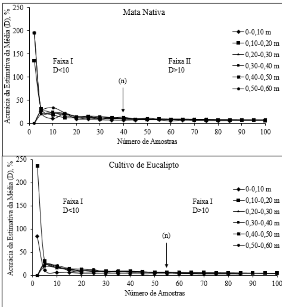
Figura 3. Precisão da estimativa das médias de resistência do solo à penetração de um Latossolo Vermelho Eutroférico em função do número de amostras /pontos coletados, para área total de 19 ha. *(n) número de amostras representativas para médias de resistência do solo à penetração. Palmeiras de Goiás, 02/2014.
