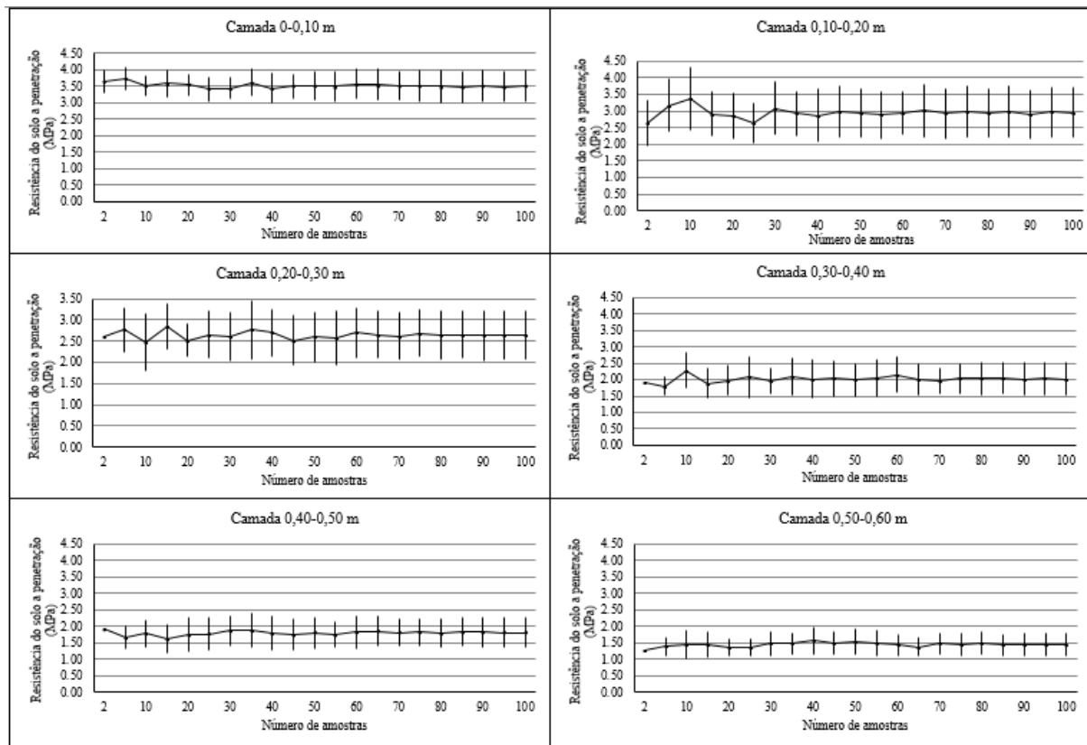
Figura 2. Variação dos valores de resistência do solo à penetração e os respectivos desvios padrões de um Latossolo Vermelho Distrófico sob cultivo de eucalipto (1 ano) em função da população amostral (n), para área total de 19 ha. Palmeiras de Goiás, 02/2014.
